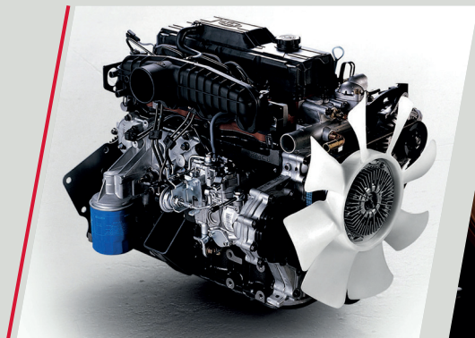
Motor 2.5 L Turbodiesel Intercooler 16 Válvulas. Potência máxima: 130,5 cv / 3.800 rpm - Torque máximo: 26 Kgm / 1.500 rpm
